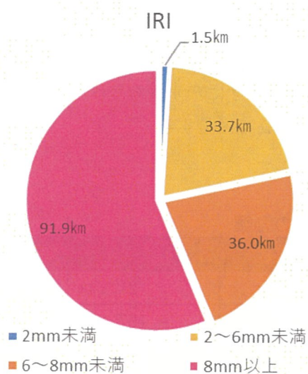
図-1.3 路面性状調査結果のまとめ
